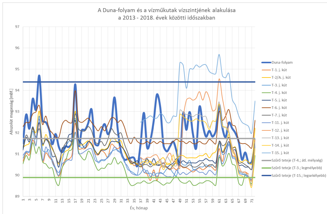
6. ábra: A Duna és a vízműkutak nyugalmi vízszintjének alakulása 2013-2018. között (a szerző saját szerkesztése)
