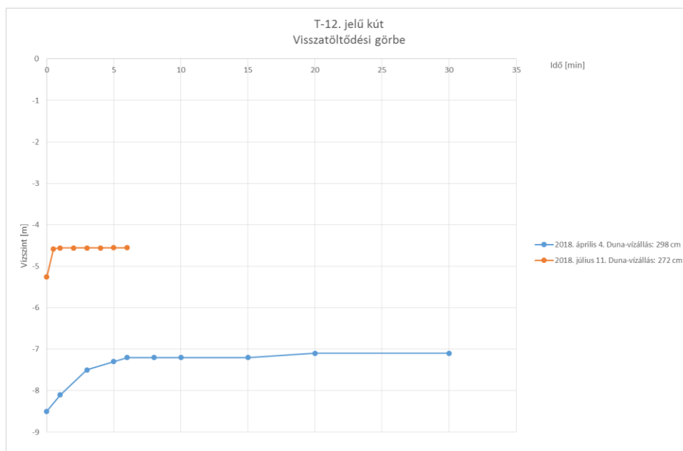
9 és 10. ábra: A karbantartási munka eredményességének ellenőrzését szolgáló Q – H, illetve visszatöltődési görbe (a szerző saját szerkesztése)
