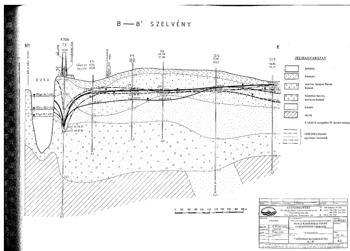
5. ábra: A vízbázis vízföldtani keresztmetszése a T-3. jelű kútnál (Geohidroterv Kft., 2001.)
