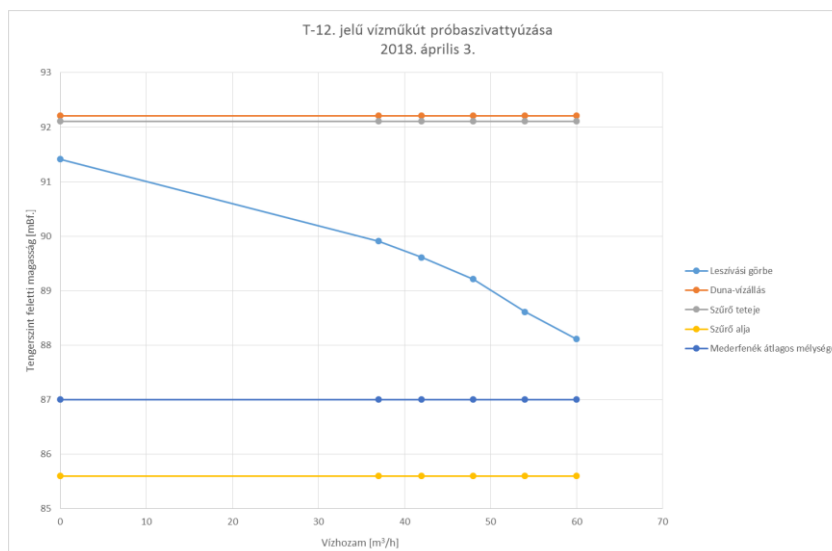
9. ábra: T-12. jelű kút Q - H görbéje (a szerző saját szerkesztése)
